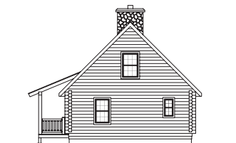
RIGHT ELEVATION
